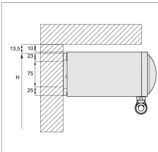
Abb. 4: notwendiger Montageaum nach oben bei Überdachungen (alle Maßangaben in mm)
